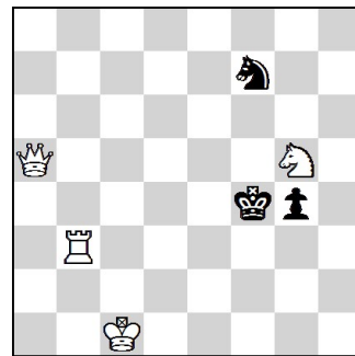
11. #2 4 + 3
